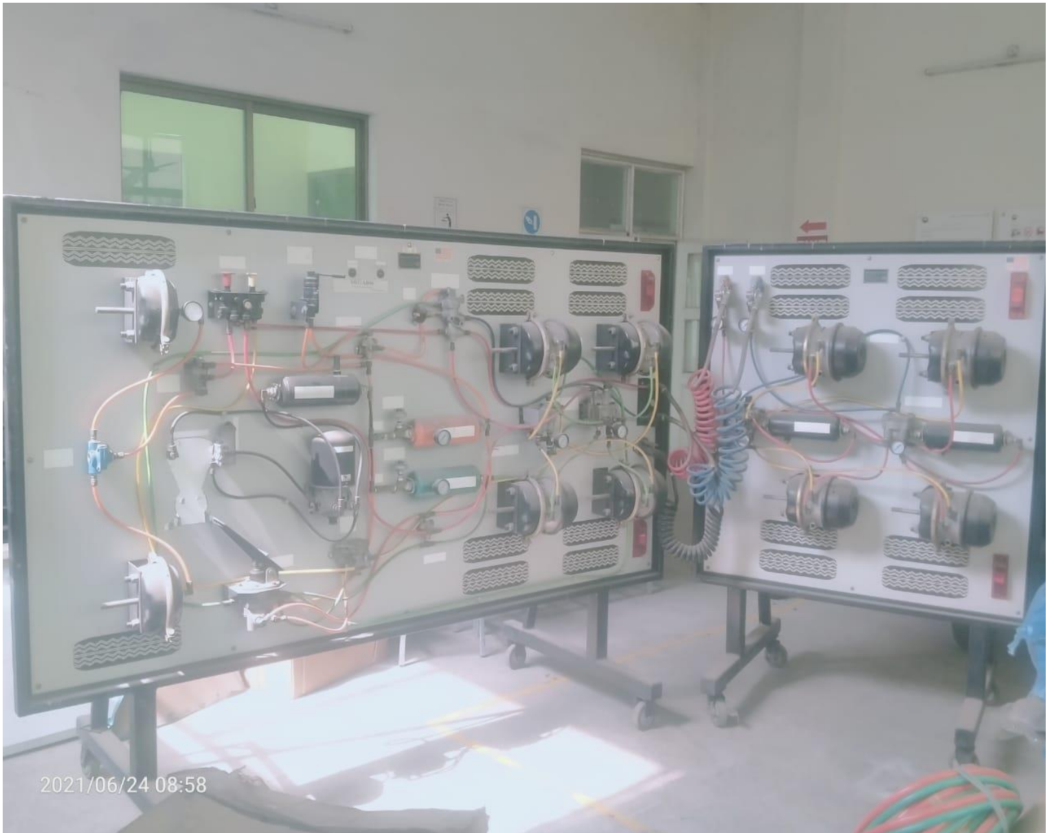
Truck Air Brake Trainer
